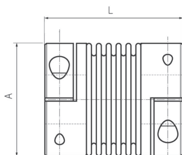
Metalbælgkobling
